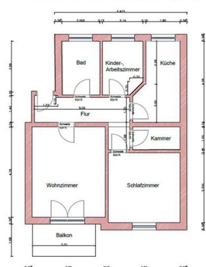
Grundriss zur Grundflächenermittlung Whg 101
